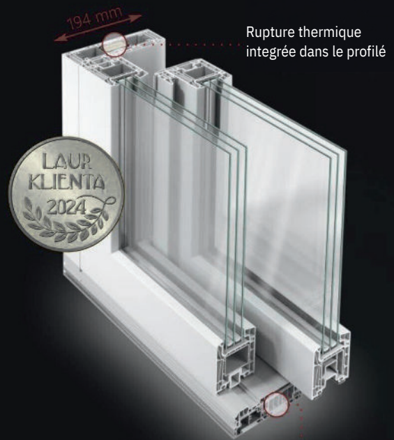
Rupture thermique intégrée dans le seuil
